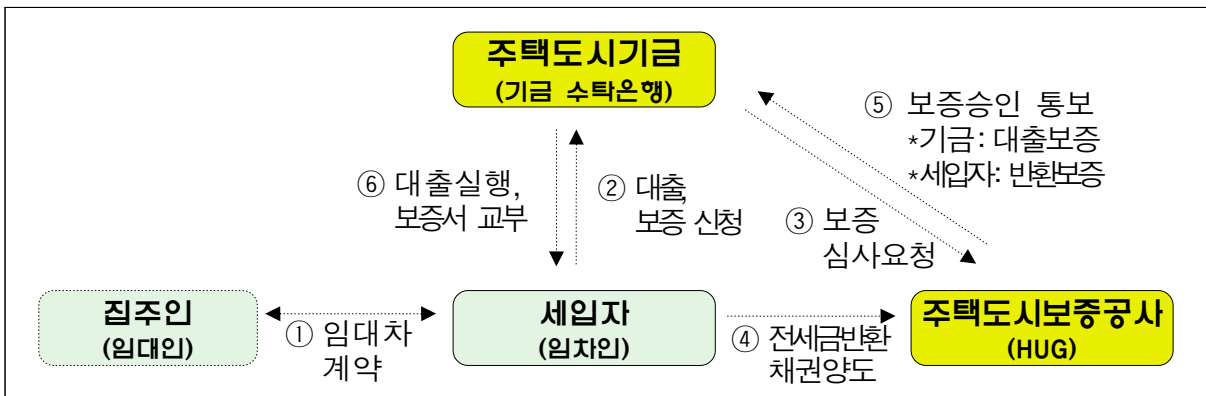
< 업무 구조도 >
